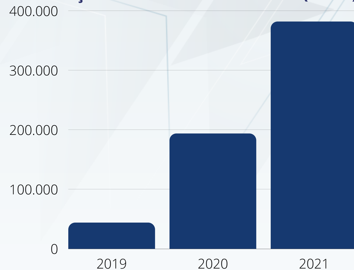
Geração Fotovoltaica anual (kWh)
